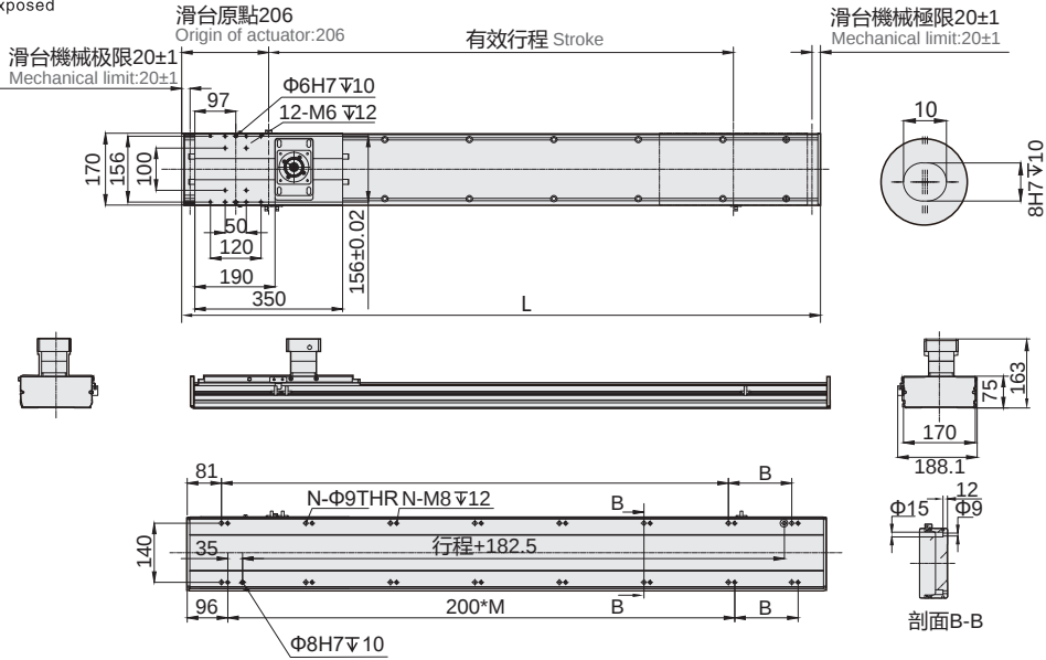
BC-A1 馬達外露 Motor Exposed
